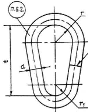
Рис. П.1.10. Звено типа У
