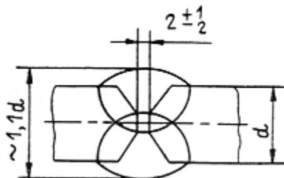
Рис. 3. Конструктивные элементы шва сварного соединения
