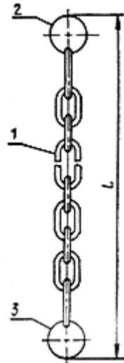
Рис. П.1.27. Одноветвевой строп: 1 - цепная ветвь, 2 - звено, 3 - захват
