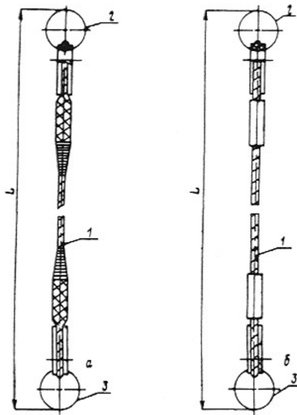
Рис. П.1.21. Одноветевой строп (а - заделка концов каната заплеткой, б - опрессовкой алюминиевой втулкой): 1 - канатная ветвь, 2 - звено, 3 - захват
